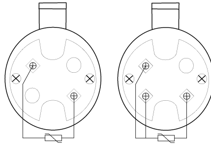
UKŁAD POŁĄCZEŃ GŁ. TYP MA POŁ. 2-PRZEWODOWE POŁ. 3-PRZEWODOWE
