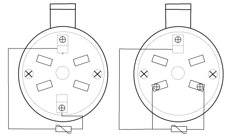
POŁ. 4-PRZEWODOWE
